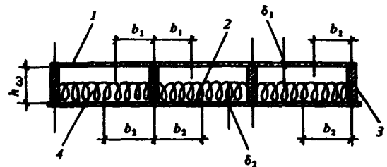
Черт 2 Поперечное сечение каркасной плиты 1,2 — асбестоцементные обшивки, 3 — элементы каркаса плиты, 4 — утеплитель
