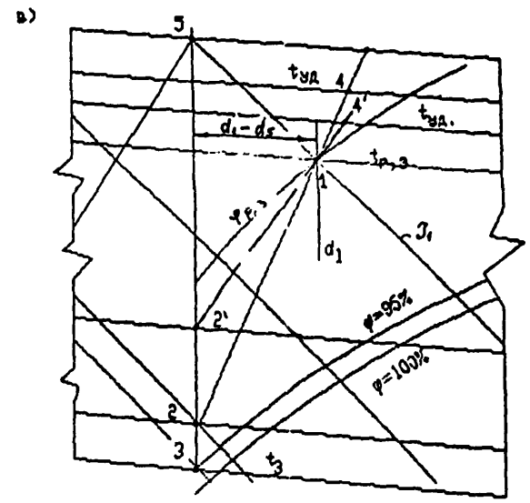
Рис. 1. Схемы процессов приготовления приточного воздуха, построение на T - d диаграмме: а - по адиабатному процессу, б - по политропному процессу, в - по политропному процессу с применением доувлажнения воздуха в помещении.
