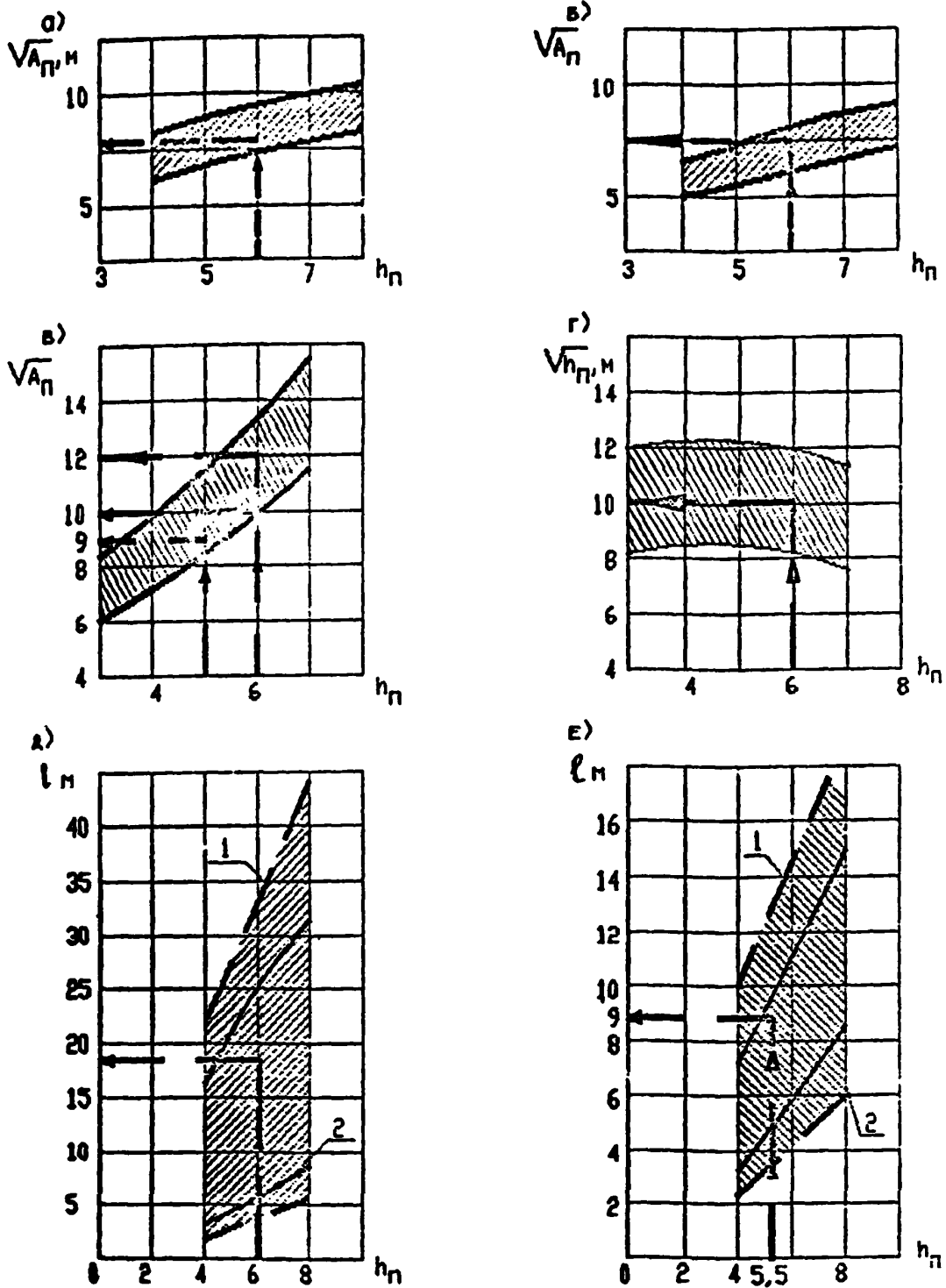
Рис. 3. Максимальный размер помещения или его зоны l = \sqrt{A_n} , м; A_n - площадь помещения или его зоны, обслуживаемая одним воздухоораспределителем, \text{м}^2 ; а - компактной струей из плоского, рис. 2г, при m = 1, 1 ; б - то же, при m = 3, 6 ; в - веерной струей, рис. 2б; г - конической струей, рис. 2д; д - рас- тилующаяся струя из решетки, рис. 2ж, при m = 6 ; 1 - ширина струи 'в' мини- мальная; 2 - ширина струи максимальная; е - растилующаяся струя из решетки при m = 2, 4 ; h_n - высота установки воздухоораспределителя.
