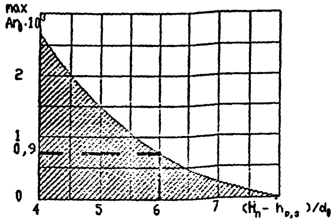
Рис. 4. ПРЕДЕЛЬНОЕ ЗНАЧЕНИЕ КРИТЕРИЯ АРХИМЕДА Ar_0 , ПРИ КОТОРОМ СОХРАНЯЕТСЯ РАСЧЕТНАЯ СХЕМА РАЗВИТИЯ СТРУИ h_n и h_{p,z} - высоты помещения и рабочей зоны, d_0 = 1,13 \cdot A_0^{0,5} , где A_0 - расчетная площадь воздухоораспределителя, m^2 , по прил. 2.
