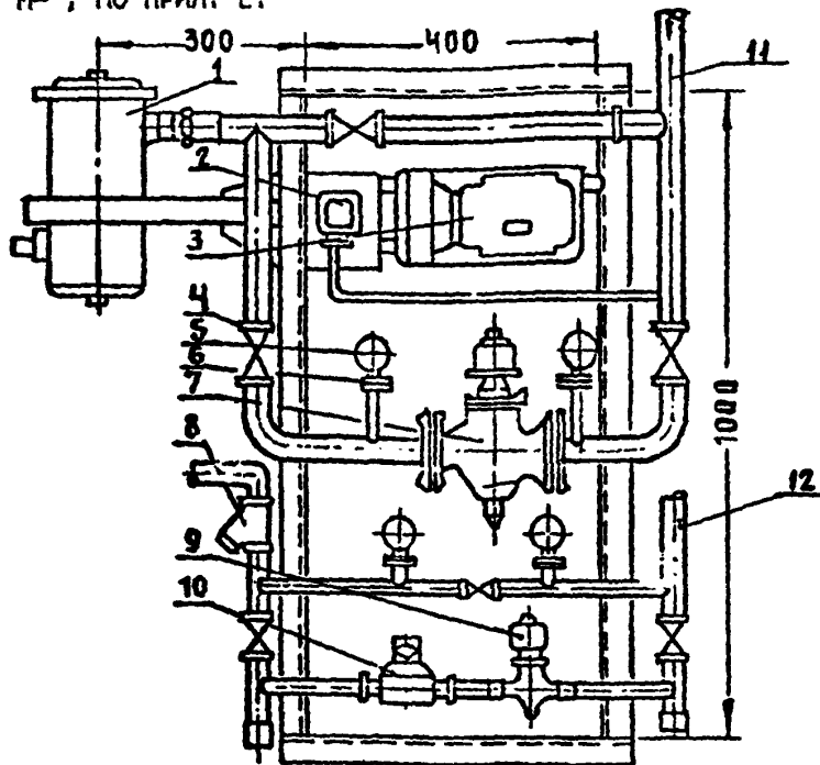
Рис. 5. ПРИМЕР КОМПОНОВКИ ШИТА УПРАВЛЕНИЯ УСТАНОВКИ 'Туман': 1 - компрессор типа МСН; 2 - реле давления РД-1-01; 3 - щиток автоматики; 4 - кран сольничковья мутовья \varnothing 32 ; 5 - манометр МТ-1; 6 - трехходовая кран КТК; 7 - вентиль СВМ \varnothing 40 ; 8 - фильтр для воды Ф-1; 9 - вентиль СВМ \varnothing 15 ; 10 - регулятор давления РДЖ-1А; 11 - трубопровод воздуха к форсунке; 12 - трубопровод воды к форсунке.
