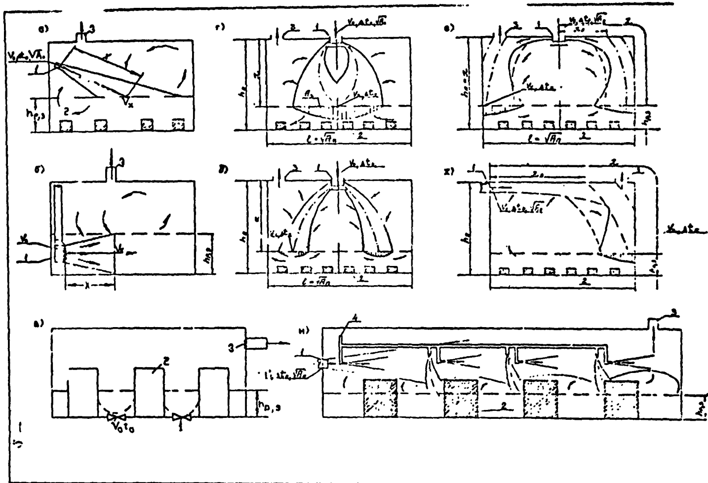
Рисунок 2. Способы подачи воздуха в производственные помещения: 1 - воздухоораспределитель; 2 - источник выделения теплоты; 3 - вытяжное устройство; 4 - воздуховод; X - расчетная длина струй приточного воздуха, м;
